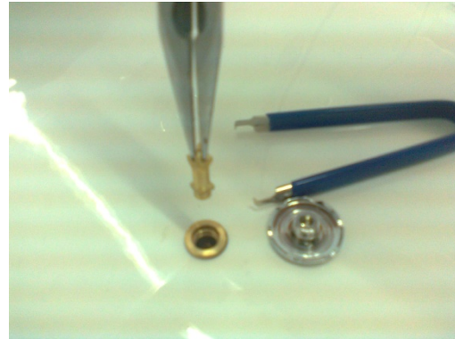
Mit einer Spitzzange oder Pinzette Rückschlagventil herausziehen
