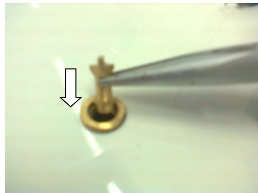
Rückschlagventil säubern, abtrocknen und mit dem runden Ende nach unten wieder einsetzen
